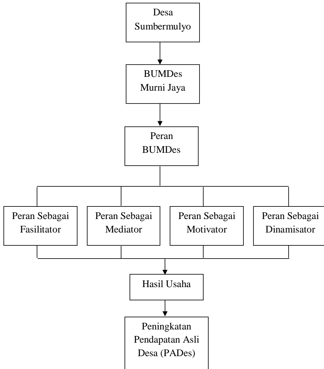
Gambar 2.1 Kerangka Konseptual
