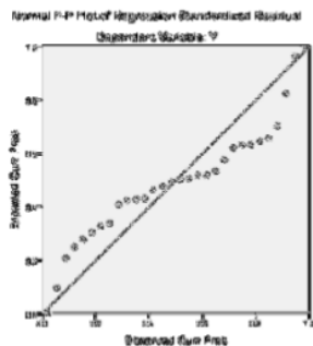
Gambar 4.1 Uji Normalitas
